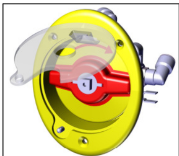
11046.00.0 GRUPPO RUBINETTO CON SCODELLINO
