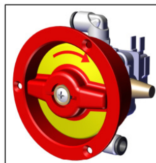
10463.00.0 MANIGLIA DI EMERGENZA ESTERNA
