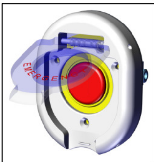
13573.00.0 GRUPPO PULSANTE DI EMERGENZA CON SPORTELLINO
