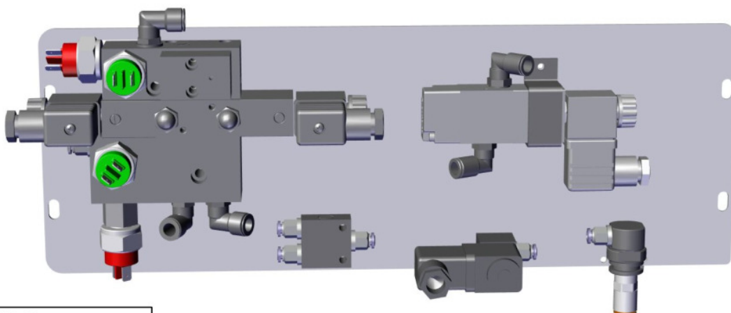
14972.00.0 GRUPPO PNEUMATICO PNEUMATIC UNIT
